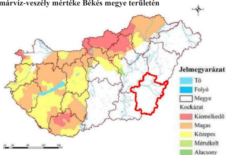
19. ábra: A villámárvíz-veszély mértéke Békés megye területén
