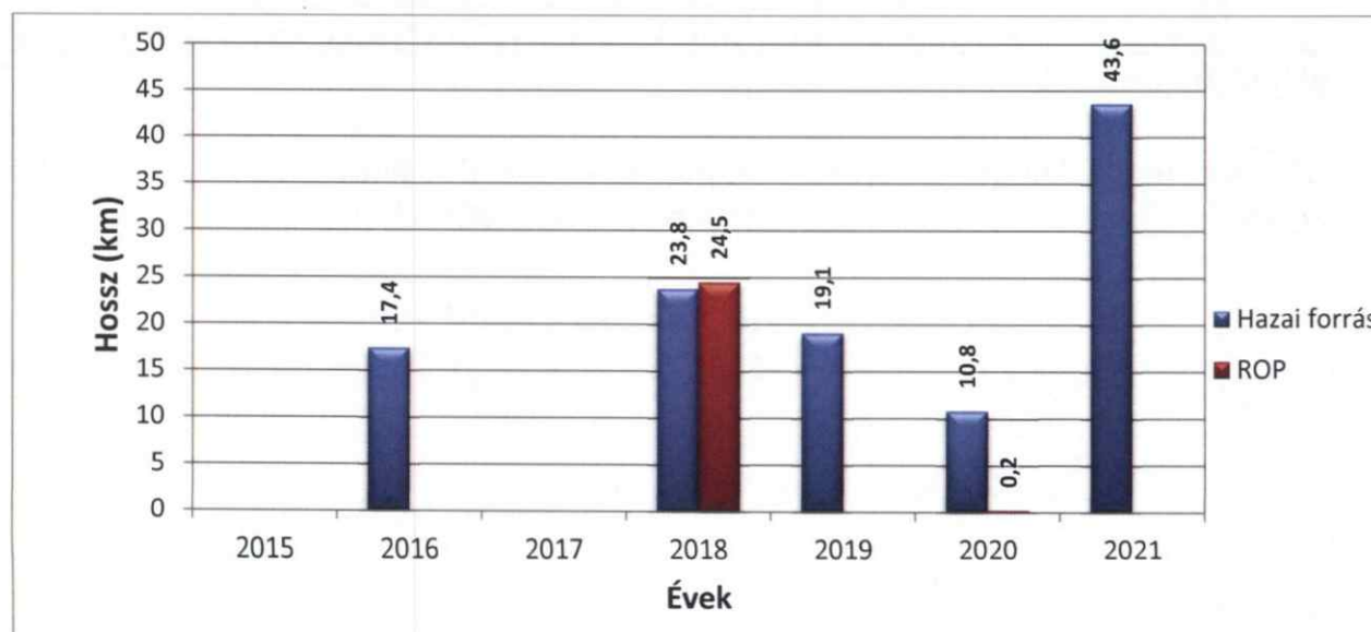
A Békés megyei útfelújítások évenkénti alakulása 2015-2021 (km)
