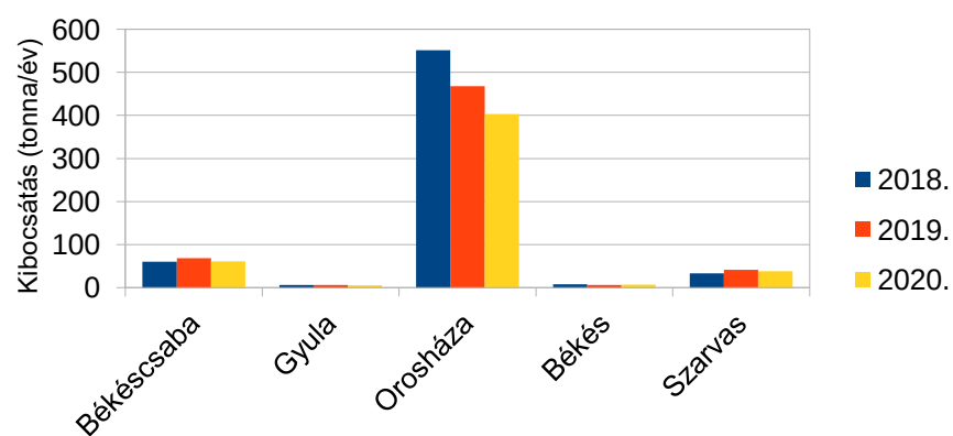
Békés megye nagyobb településeinek NOx kibocsátása
